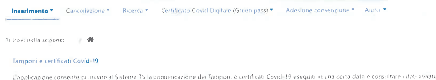
Figura 3 Funzionalità dell'applicazione
