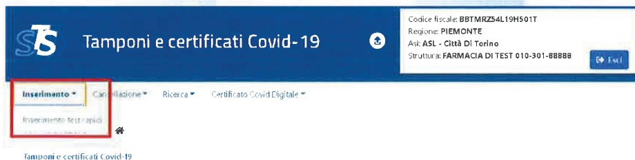
Figura 5 menu "Inserimento"
